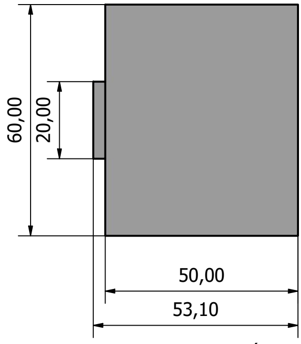
Tapa de batería
